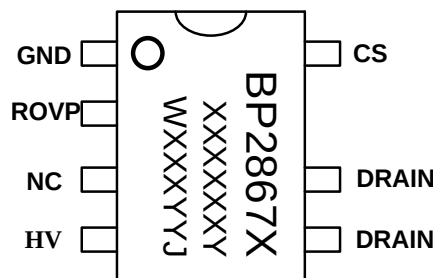
图 2 管脚封装图
