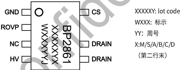
图 2 管脚封装图
